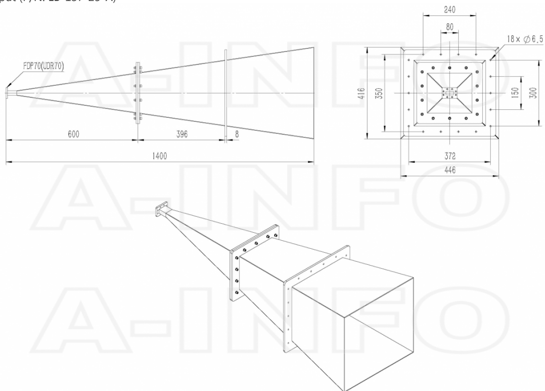
FDP70 Output (P/N: LB-137-25-A)
